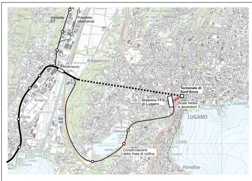
Fig. 18 Schema auspicato per l'infrastruttura Tram-Treno del Luganese
