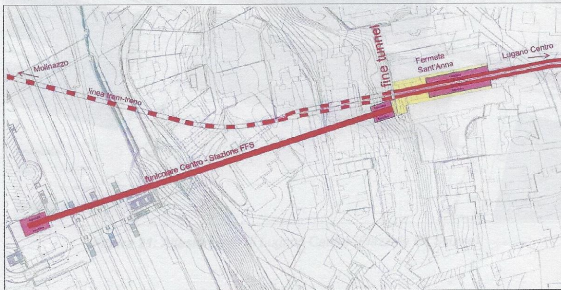
Fig. 5 Nel rapporto conclusivo del citato studio di fattibilità, del 2005, si era proposta una funicolare per la Stazione FFS, legata alla fermata di Sant'Anna.
