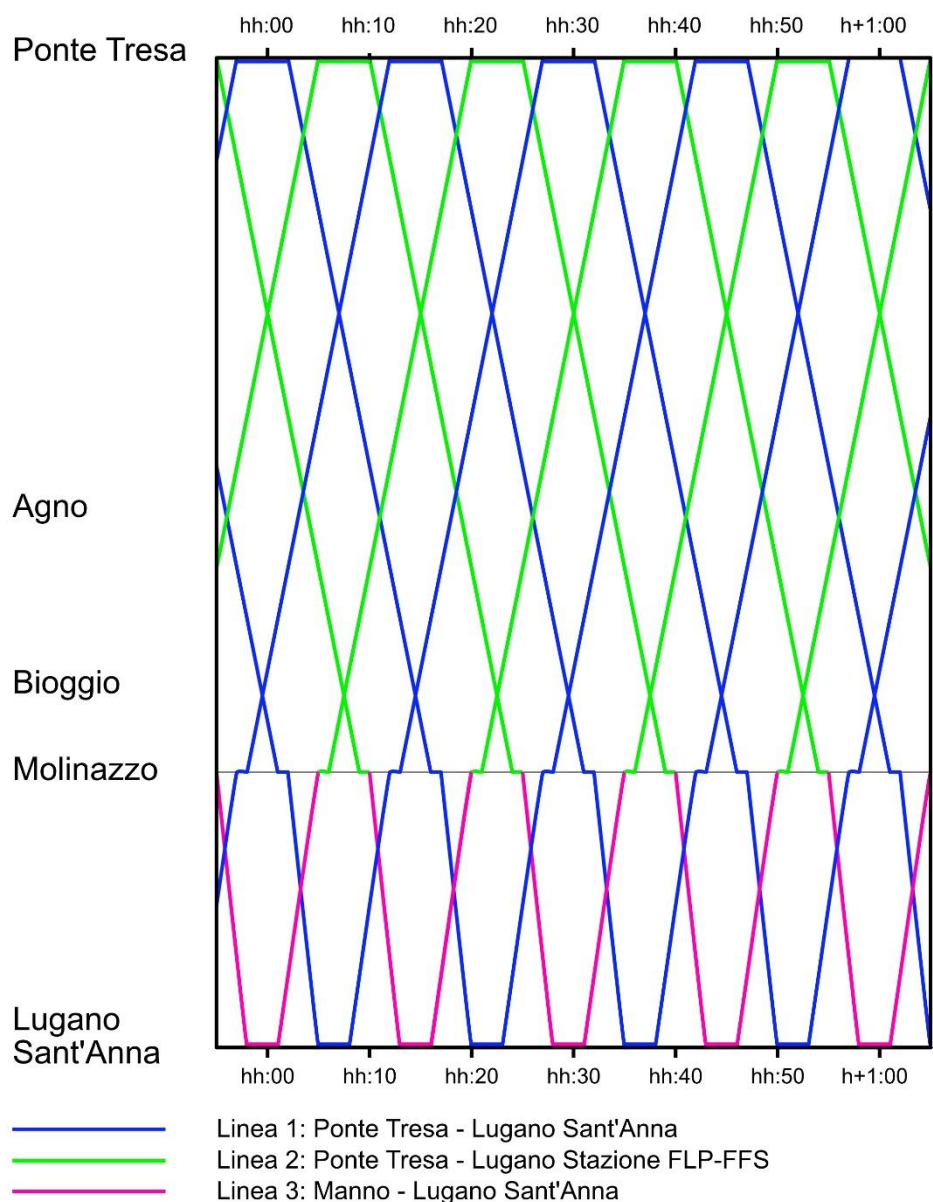
Fig. 16 Orario grafico della proposta d'orario
