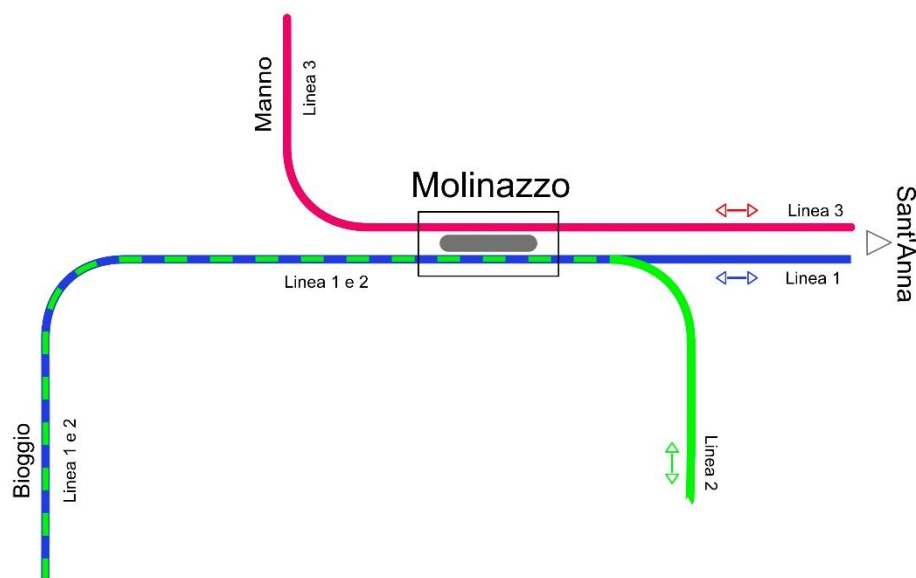
Fig. 17 Schema dei binari e dell'esercizio prospettato
